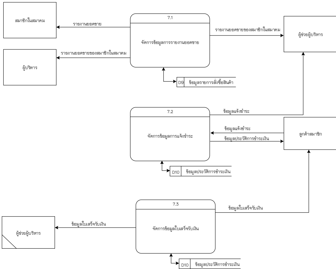
ภาพที่ 3.5 แสดงแผนภาพกระแสข้อมูลระดับที่ 1 จัดการข้อมูลผู้ใช้ระบบ
